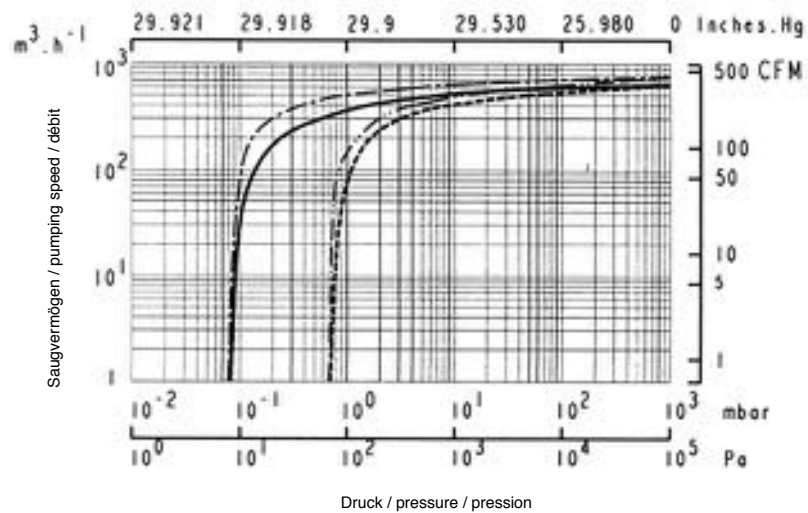
Fig 2 Saugvermögenskurven Pumping speed (volumen flow rate) Courbes de débit SV 630 ——— ohne Gasballast without gas ballast sans lest d'air SV 630 - - - - mit Gasballast with gas ballast avec lest d'air SV 750 ——— ohne Gasballast without gas ballast sans lest d'air SV 750 - - - - mit Gasballast with gas ballast avec lest d'air
