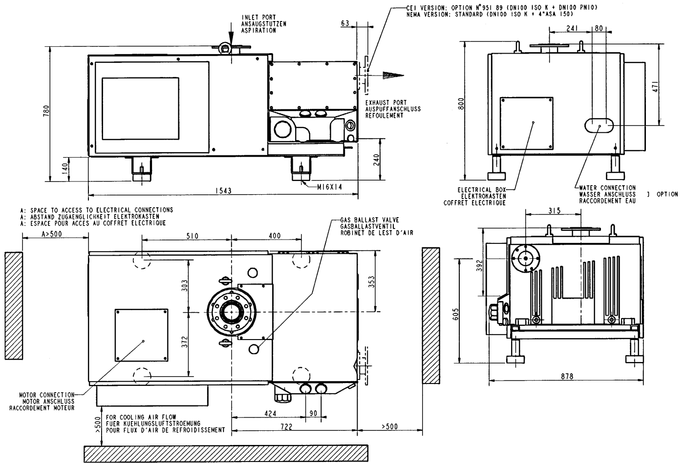
Fig 1 Maßzeichnung Dimensional drawing Plan d'encombrement
