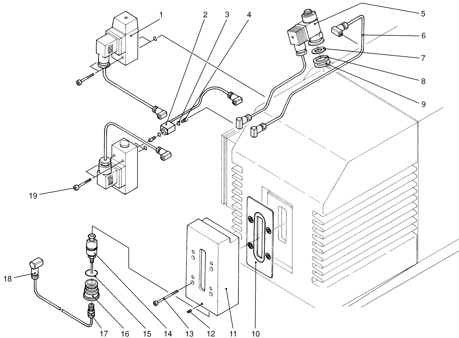
Abb. / Fig. 1 LSS 40-65; LSS 16-25 ähnlich/similar/similaire
