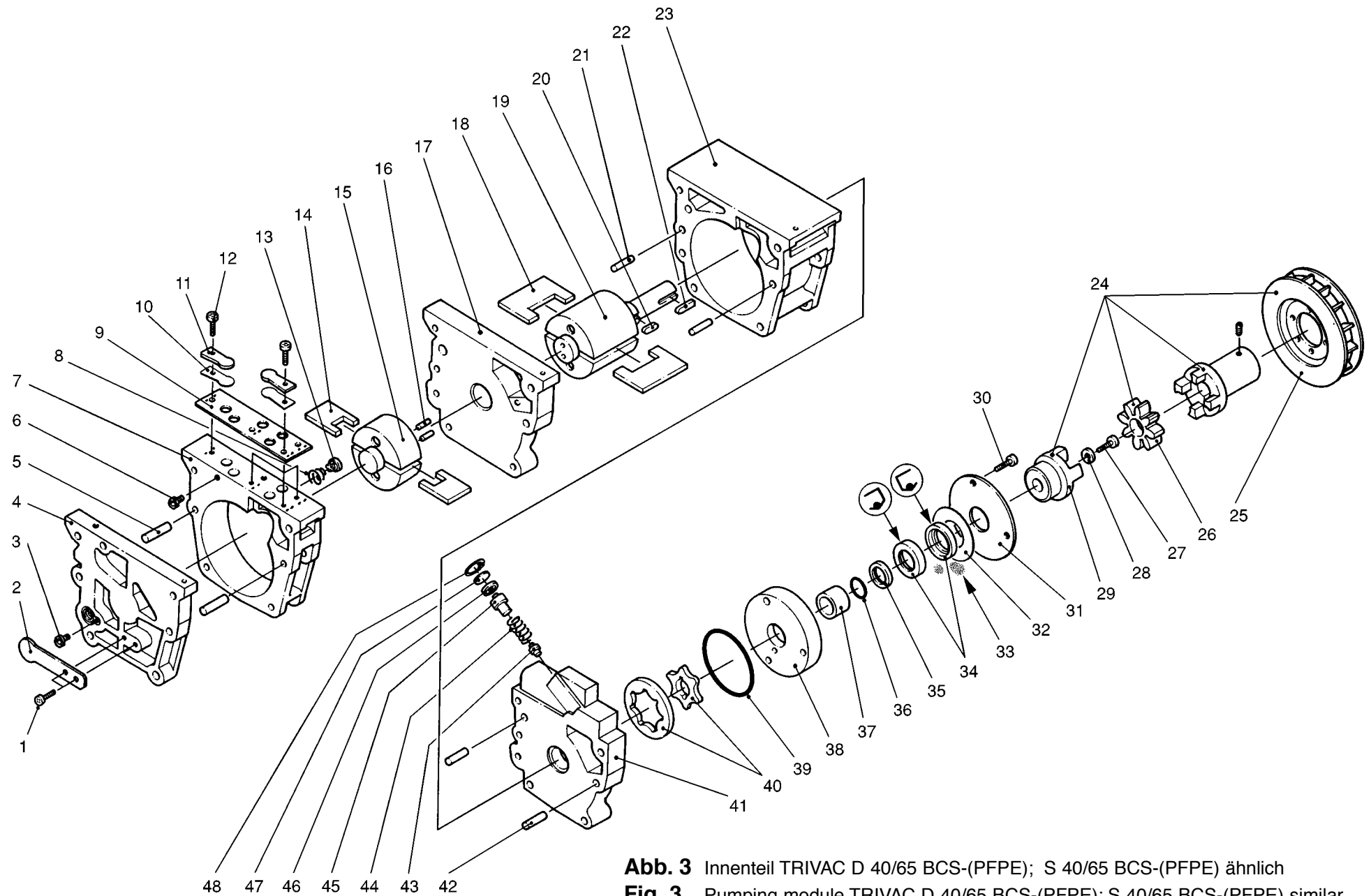
Fig. 3 Corps de pompe TRIVAC D 40/65 BCS-(PFPE); S 40/65 BCS-(PFPE) similaire
