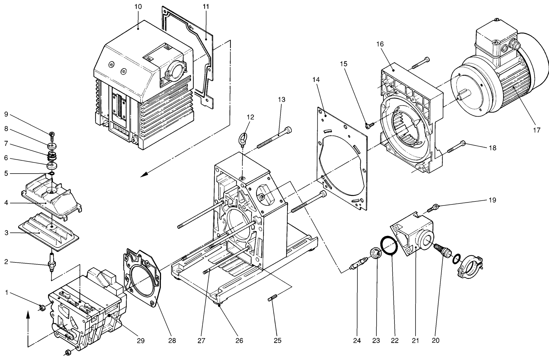
Abb./Fig. 2 TRIVAC D 40/65 BCS-(PFPE); S 40/65 BCS-(PFPE) ähnlich/similar/similaire
